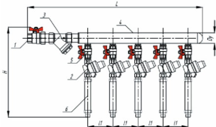
Коллекторный узел ХВС и ГВС с индивидуальным регулятором (Вариант 3)
