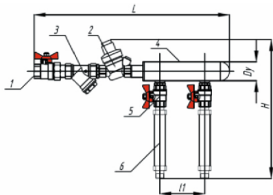
Коллекторный узел ХВС и ГВС с общим регулятором (Вариант 1)
