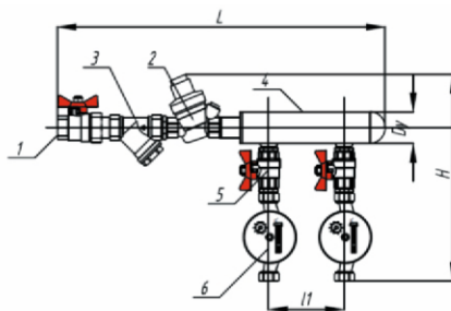
Коллекторный узел ХВС и ГВС с общим регулятором и счетчиками (Вариант 2)
